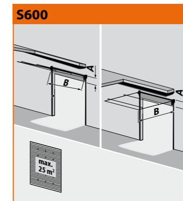
Helix S600 Horizontaal railsysteem
