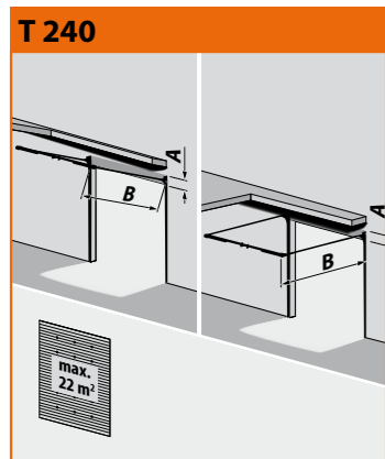
T 240 Laaginbouw railsysteem, binnenliggende kabels + stalen draagprofiel
