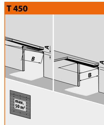
T 450 Normaal railsysteem (standaard)
