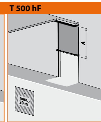
T 500 hF Verticaal railsysteem met laagliggende veeras + stalen draagprofiel
