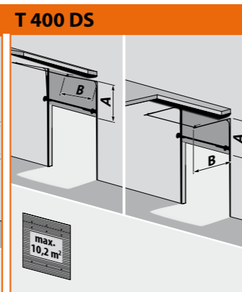
T 400 DS Verhoogd railsysteem met laagliggende veeras
